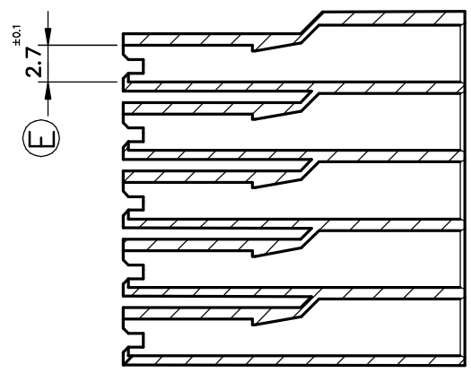
Sección B-B
