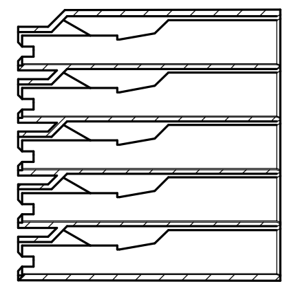
Sección A-A
