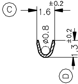
SECC. B-B'
