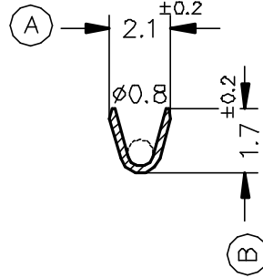
SECC. A-A'
