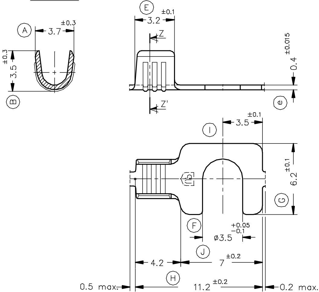
Secc. Z-Z'
