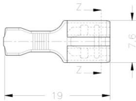
Secc. Z-Z
