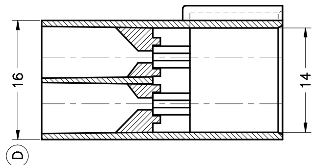
Secc. A-A
